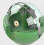
Die „Rattenkugel“ (auch digital): Bei Rückstau schwimmt die Rattenkugel am Aufhängungsseil auf und ab und senkt sich nach dem Rückstau wieder.
